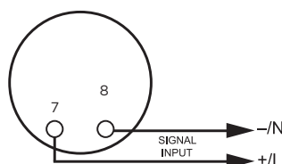
FIG. AA 007-05/007-41
